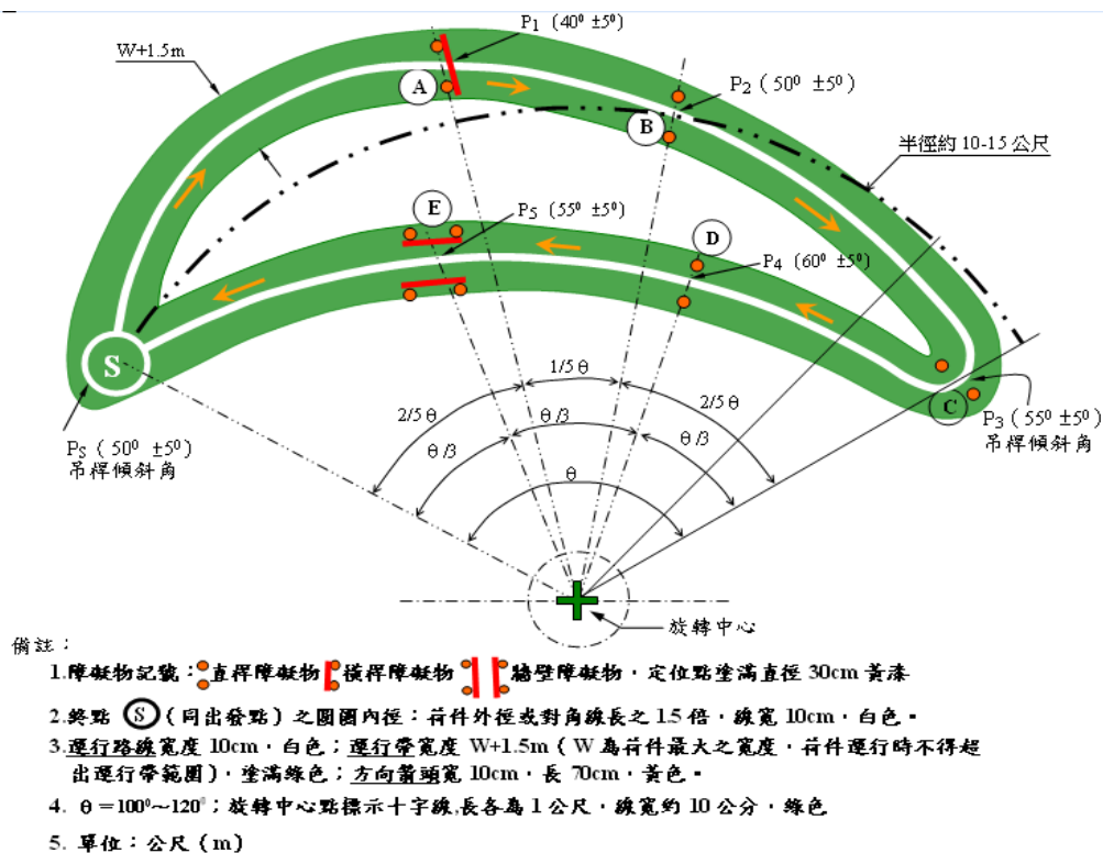
附圖一 移動式(伸臂不伸縮)起重機荷物吊運路線圖
